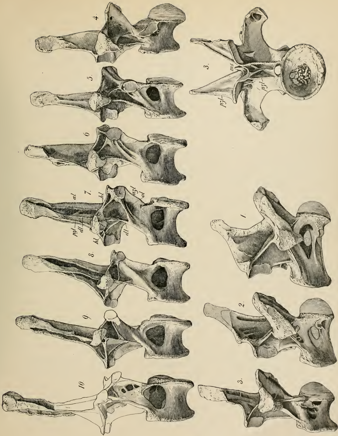
ANTERIOR DORSALS OF DIPLODOCUS CARNEGII HATCHER (No. 84). \frac{1}{16} NAT. SIZE.
